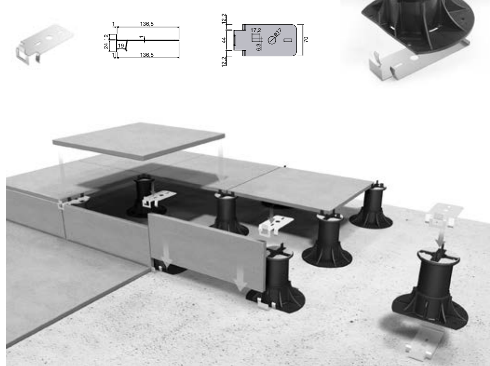
TOP VERTICAL EDGE CLIP
